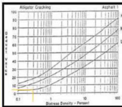
Gambar 2.22 Deduct value retak kulit buaya. (Sumber : Shahin, 1994)
