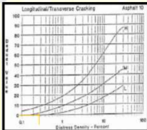
Gambar 2.31 Deduct value retak memanjang/melintang. (Sumber : Shahin, 1994)
