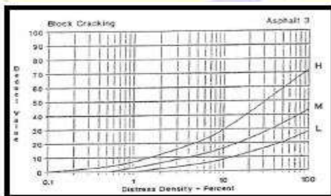
Gambar 2.25 Deduct value retak kotak-kotak. (Sumber : Shahin, 1994)
