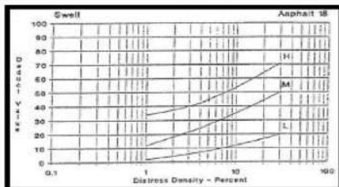
Gambar 2.37 Deduct value mengembang jembul. (Sumber : Shahin, 1994)
