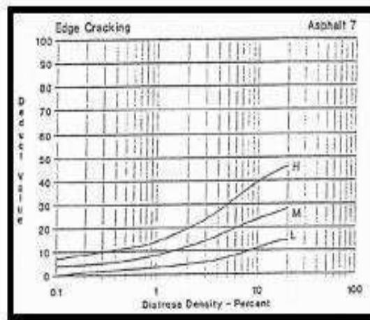
Gambar 2.28 Deduct value retak pinggir jalan. (Sumber : Shahin, 1994)
