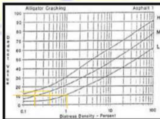
Gambar 2.22 Deduct value retak kulit buaya. (Sumber : Shahin, 1994)
