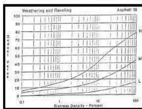
Gambar 2.37 Deduct value pelepasan butir. (Sumber : Shahin, 1994)
