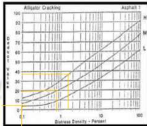
Gambar 2.22 Deduct value retak kulit buaya. (Sumber : Shahin, 1994)
