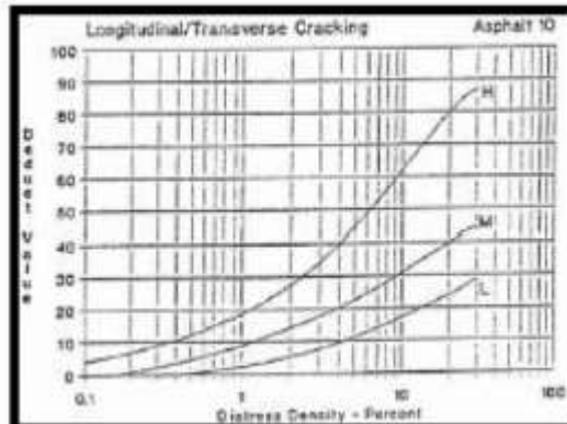
Gambar 2.37 Deduct value pelepasan butir. (Sumber : Shahin, 1994)
