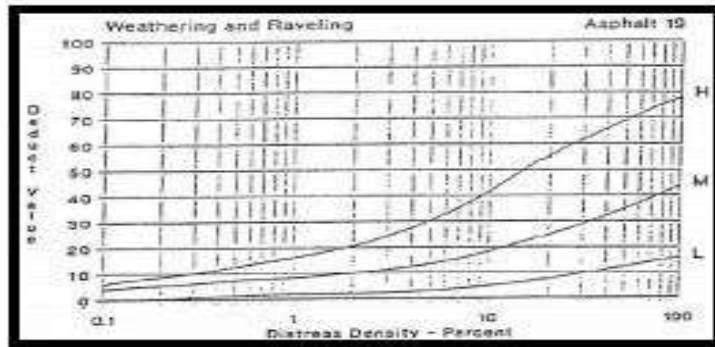
Gambar 2.38 Deduct value permukaan butir. (Sumber : Shahin, 1994)
