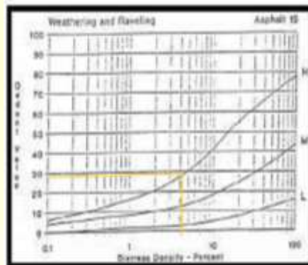
Gambar 2.37 Deduct value pelepasan butir. (Sumber : Shahin, 1994)
