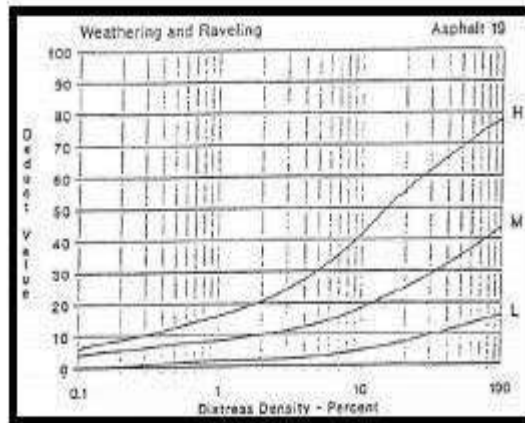
Gambar 2.37 Deduct value pelepasan butir. (Sumber : Shahin, 1994)
