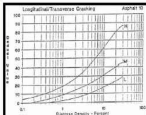
Gambar 2.31 Deduct value retak memanjang/melintang. (Sumber : Shahin, 1994)
