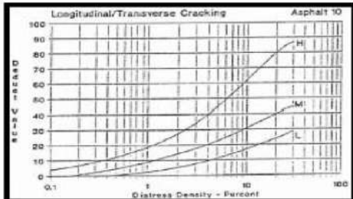
Gambar 2.32 Deduct value retak memanjang/melintang. (Sumber : Shahin, 1994)
