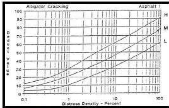
Gambar 2.23 Deduct value retak kulit buaya. Sumber : Shahin, 1994
