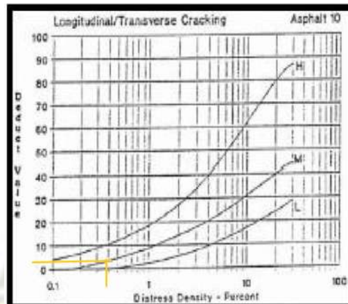
Gambar 2.31 Deduct value retak memanjang/melintang. (Sumber : Shahin, 1994)
