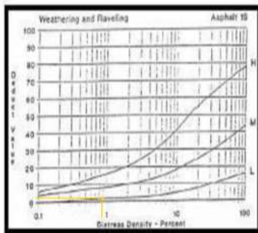
Gambar 2.37 Deduct value pelepasan butir. (Sumber : Shahin, 1994)
