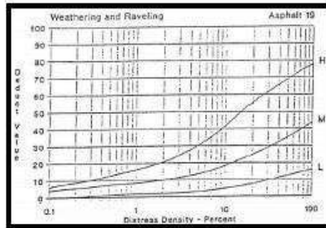
Gambar 2.31 Deduct value retak memanjang/melintang. (Sumber : Shahin, 1994)
