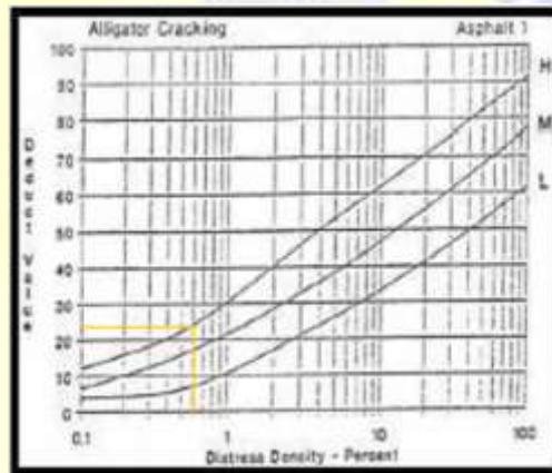
Gambar 2.22 Deduct value retak kulit buaya. Sumber : Shahin, 1994
