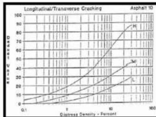
Gambar 2.31 Deduct value retak memanjang/melintang. (Sumber : Shahin, 1994)
