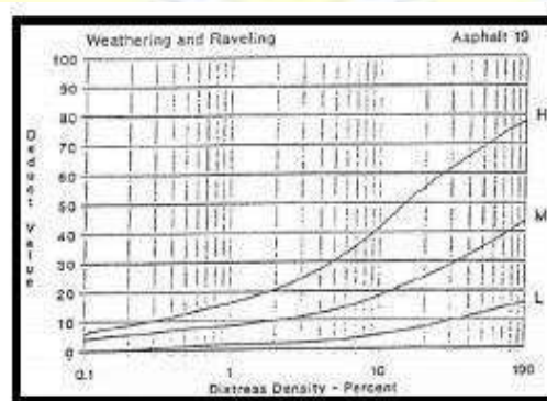
Gambar 2.31 Deduct value retak memanjang/melintang. (Sumber : Shahin, 1994)
