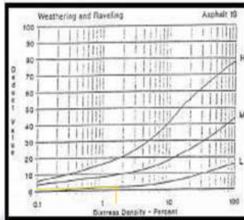
Gambar 2.37 Deduct value pelepasan butir. (Sumber : Shahin, 1994)
