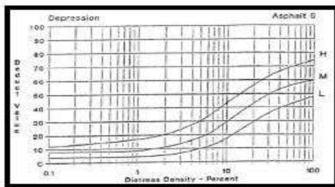
Gambar 2.28 Deduct value amblas. (Sumber : Shahin, 1994)
