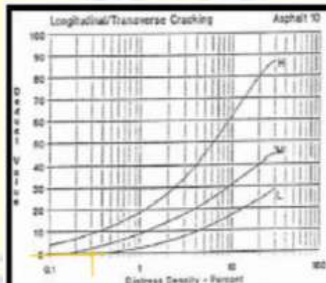
Gambar 2.31 Deduct value retak memanjang/melintang. (Sumber : Shahin, 1994)
