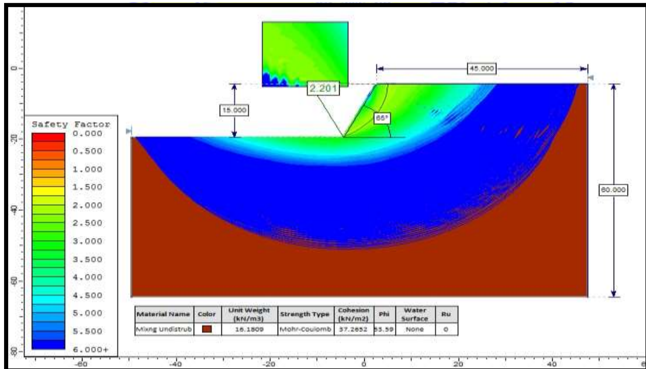
Analisis Kestabilan lereng tunggal pada kondisi kering dengan material Mixing Undistrub tinggi jenjang 15 meter sudut 65° dengan FK 2.201
