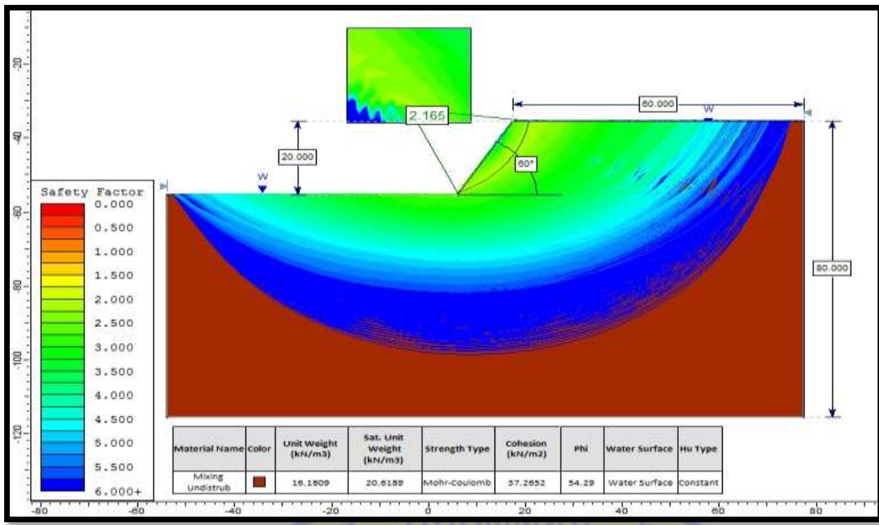
Analisis Kestabilan lereng tunggal pada kondisi setengah jenuh dengan material Mixing Undisturb tinggi jenjang 20 meter sudut 60° dengan FK 2.165
