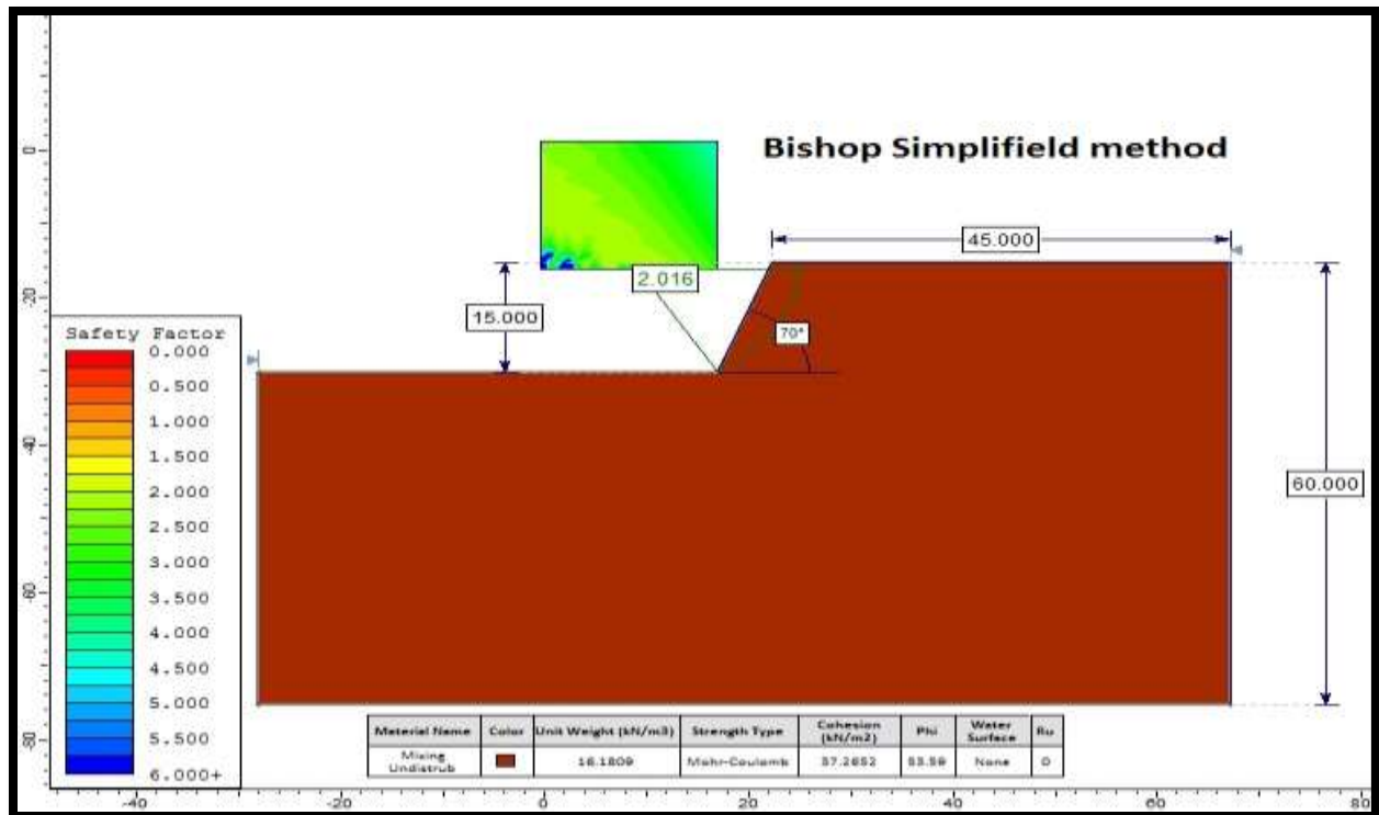
Analisis Kestabilan lereng tunggal pada kondisi kering dengan material Mixing Undisturbed tinggi jenjang 15 meter sudut 70° dengan FK 2.016
