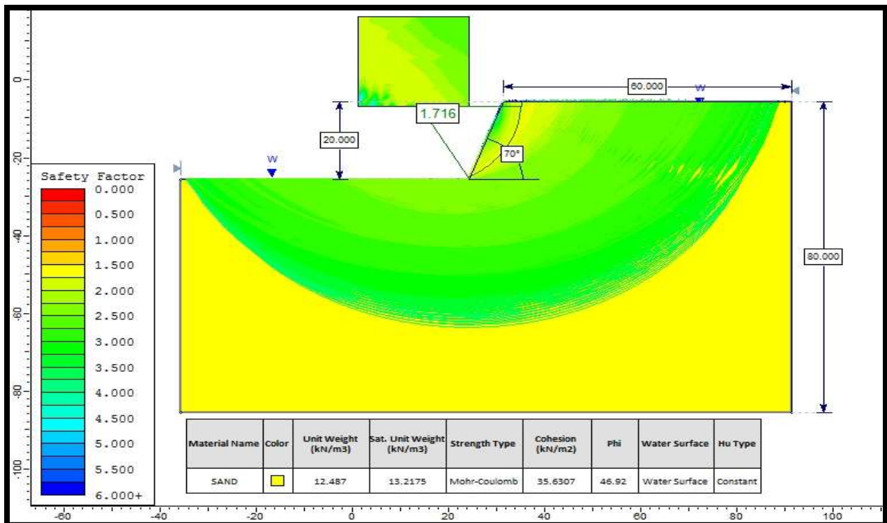
Analisis Kestabilan lereng tunggal pada kondisi setengah jenuh dengan material SAND tinggi jenjang 20 meter sudut 70° dengan FK 1.716
