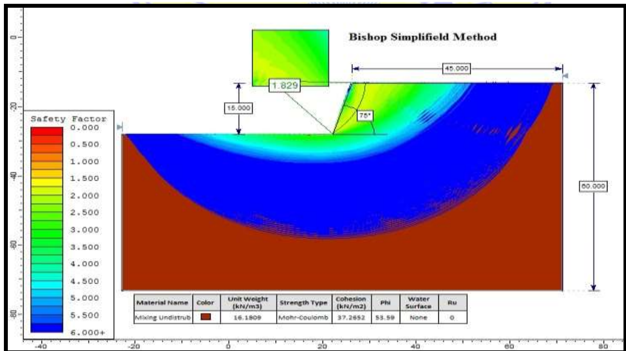
Analisis Kestabilan lereng tunggal pada kondisi kering dengan material Mixing Undisturb tinggi jenjang 15 meter sudut 75° dengan FK 1.829
