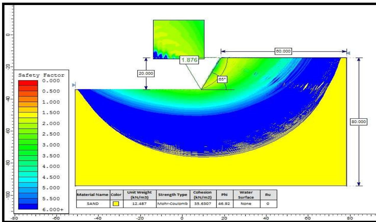
Analisis Kestabilan lereng tunggal pada kondisi kering dengan material CLAY B tinggi jenjang 20 meter sudut 65° dengan FK 1.876
