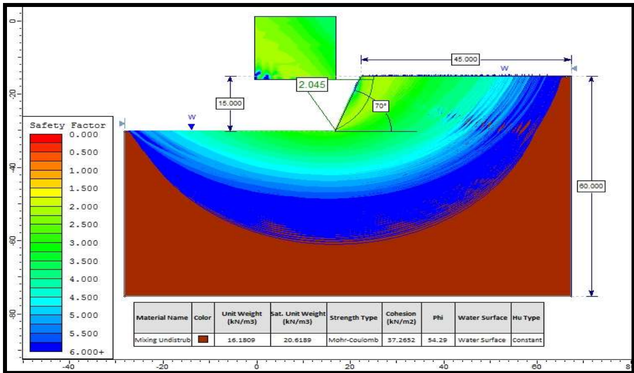
Analisis Kestabilan lereng tunggal pada kondisi setengah jenuh dengan material Mixing Undistrub tinggi jenjang 15 meter sudut 70° dengan FK 1.500
