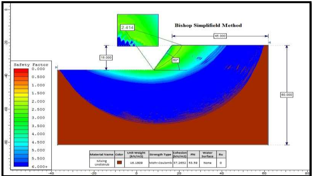
Analisis Kestabilan lereng tunggal pada kondisi kering dengan material Mixing Undistrub tinggi jenjang 15 meter sudut 60° dengan FK 2.414
