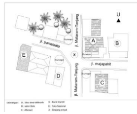
Kondisi Geometrik Simpang
