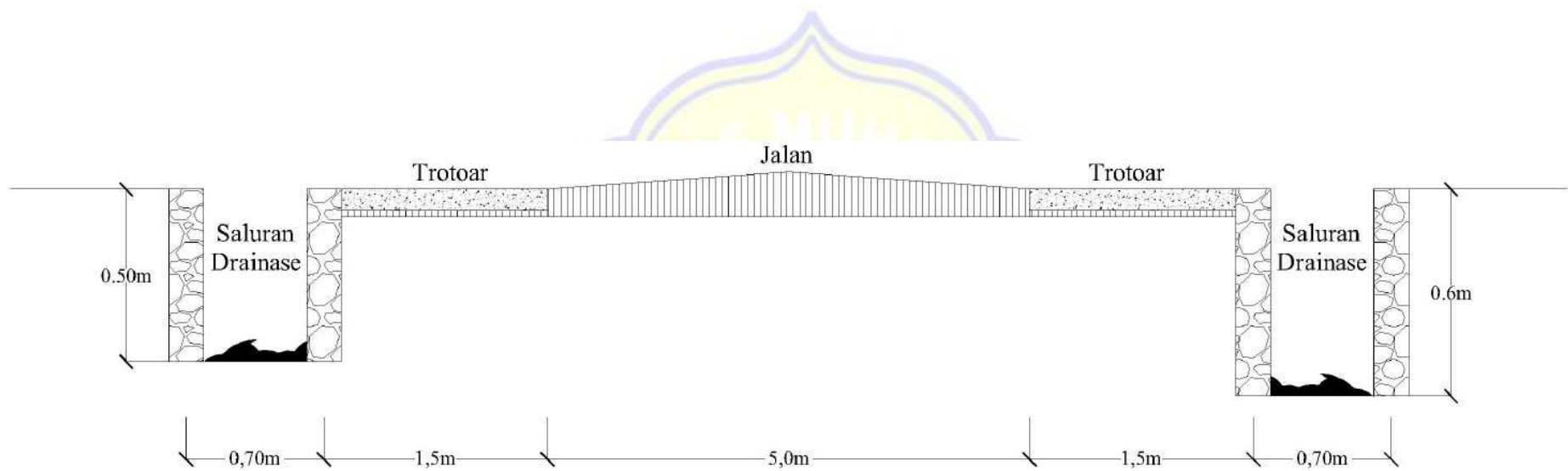
POTONGAN JALAN TITIK P-04
