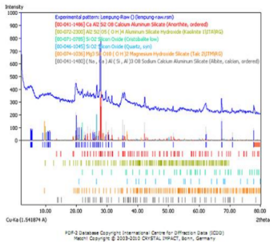
Gambar 5. Hasil Uji XRD Tanah Lempung
