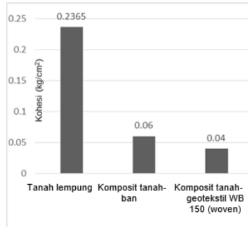
Gambar 9. Kohesi Tanah Lempung dan Komposit Tanah
