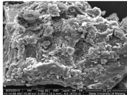
Gambar 6. Hasil Uji SEM Tanah Lempung
