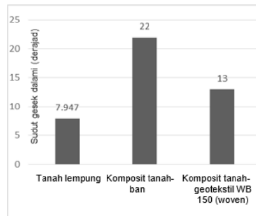
Gambar 10. Sudut Gesek Dalam Tanah Lempung dan Komposit Tanah
