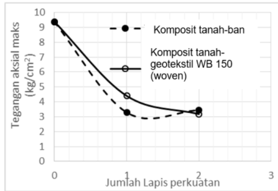
Gambar 11. Grafik Tegangan Aksial Tanah Lempung dan Komposit Tanah-ban
