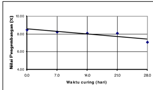
Gambar 7. Hubungan lama curing pada angka pengembangan
