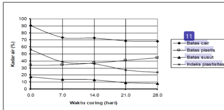
Gambar 2. Hubungan waktu curing terhadap batas-batas konsistensi
