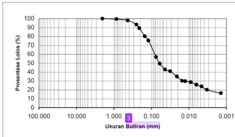
Gambar 1. Kurva Distribusi Ukuran Butiran
