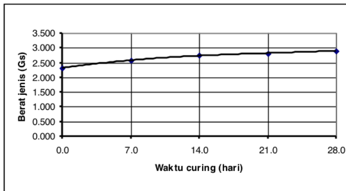
Gambar 3 Hubungan waktu curing terhadap Berat jenis (Gs)
