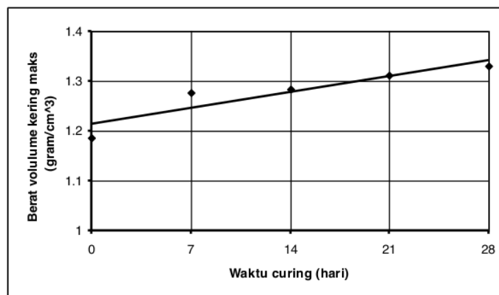
Gambar 4. Hubungan waktu curing terhadap berat volume kering maksimum
