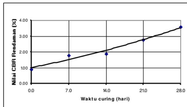
Gambar 6. Hubungan lama curing terhadap angka CBR rendaman
