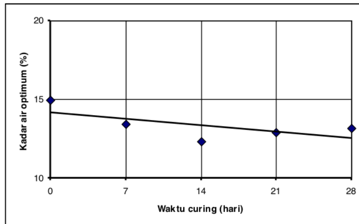
Gambar 5. Hubungan waktu curing terhadap kadar air optimum
