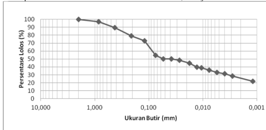
Gambar.1. Kurva Distribusi Ukuran Butiran
