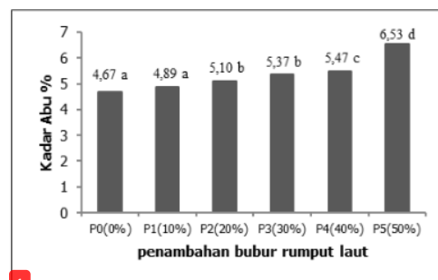
1 Gambar 2. Grafik Hubungan Pengaruh Penambahan Bubur Rumput Laut Terhadap Kadar Abu Nugget Tahu.
