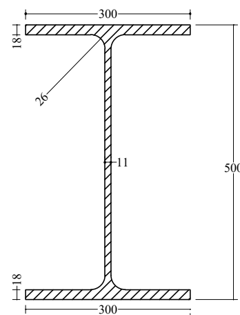
PROFIL BALOK MEMANJANG SCALA 1:10
