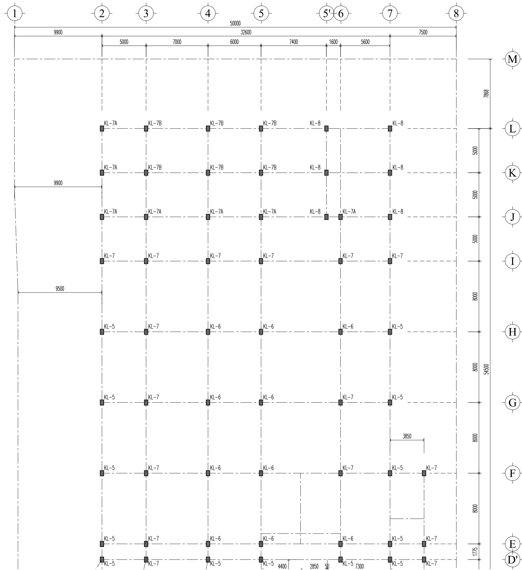
DENAH KOLOM SKALA 1:250
