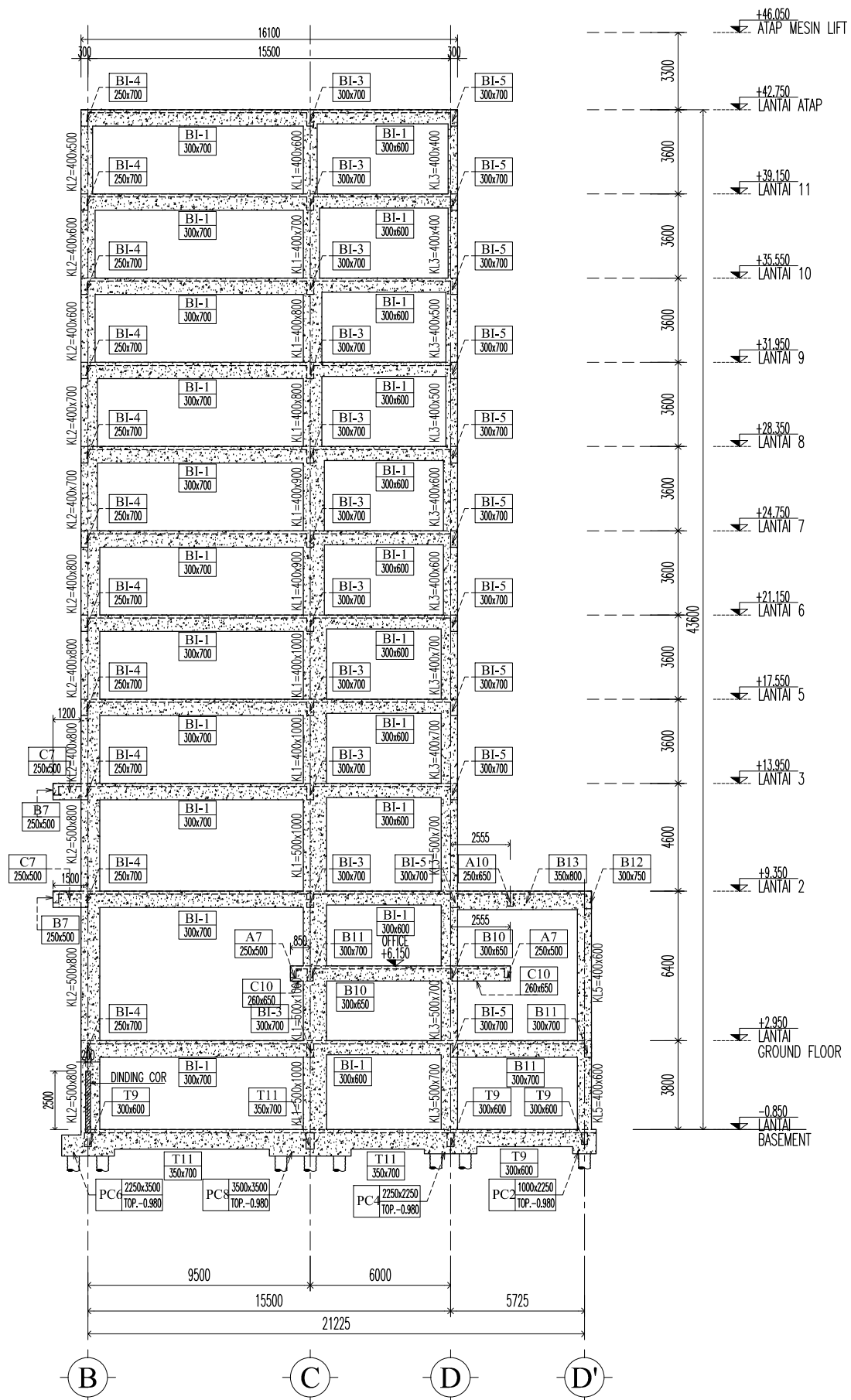
POTONGAN PORTAL T4 SKALA 1:250
