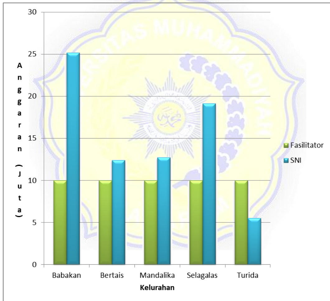
Gambar 3 Diagram perbandingan rencana anggaran biaya fasilitator dengan rencana anggaran biaya analisa SNI 2008 Kecamatan Sandubaya (Rusak Ringan)
