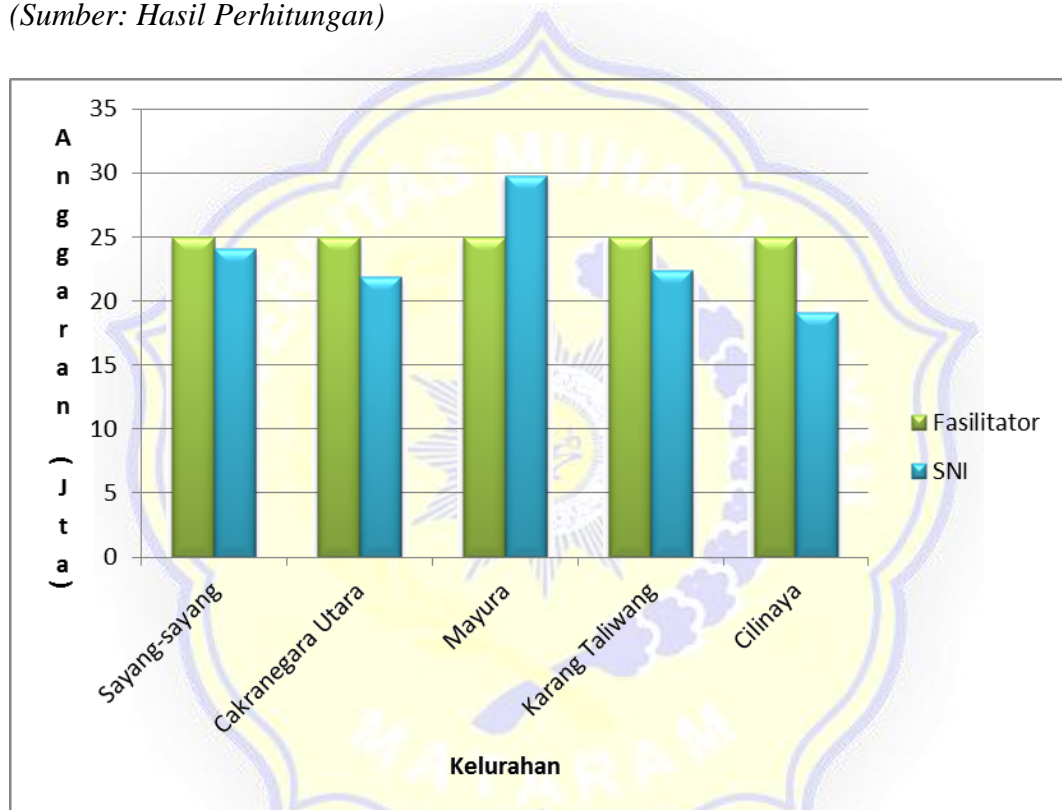
Gambar 5 Diagram perbandingan rencana anggaran biaya fasilitator dengan rencana anggaran biaya analisa SNI 2008 Kecamatan Cakranegara (Rusak Sedang)
