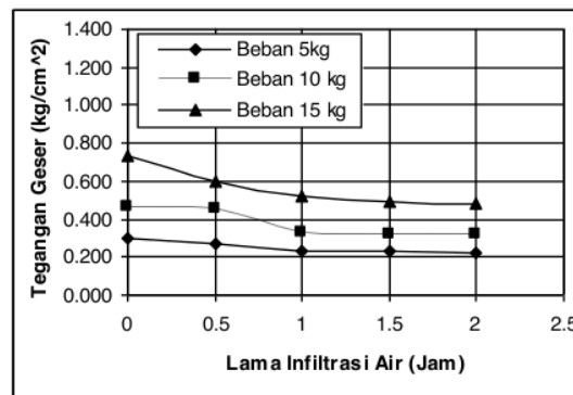
Gambar 4. Hubungan antara tegangan geser tanah dan lama infiltrasi air hujan
