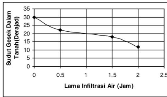
Gambar 5. Hubungan antara sudut geser dalam tanah dan lama infiltrasi air hujan
