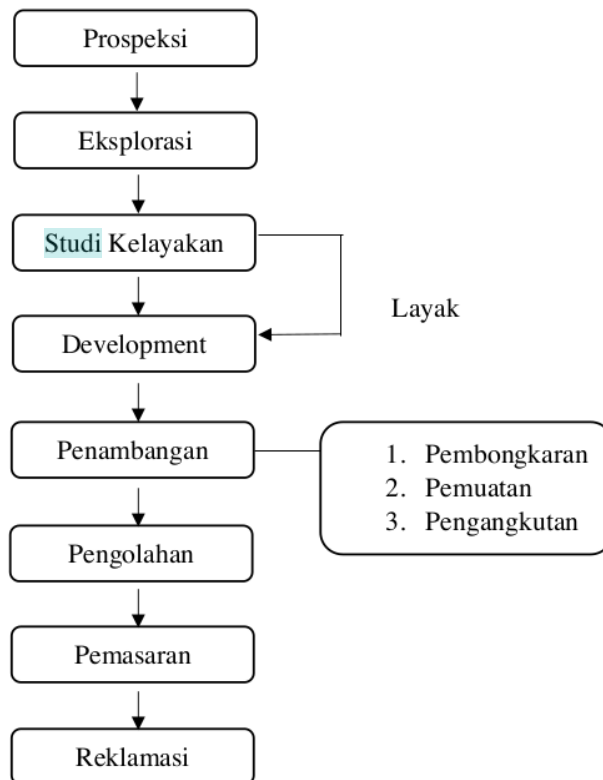
Gambar 3. 1 Diagram Alir Pertambangan
