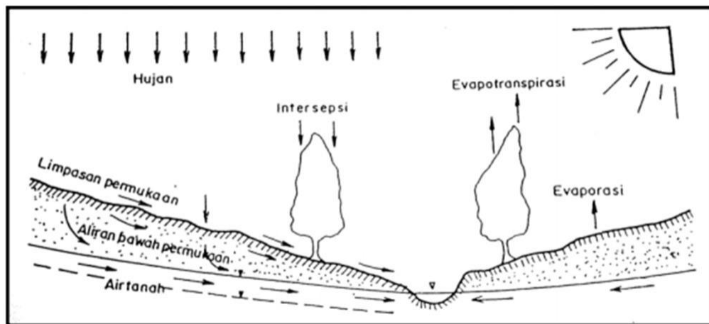
Gambar 2.1 Siklus Hidrologi (Kasiro, dkk. 1997)
