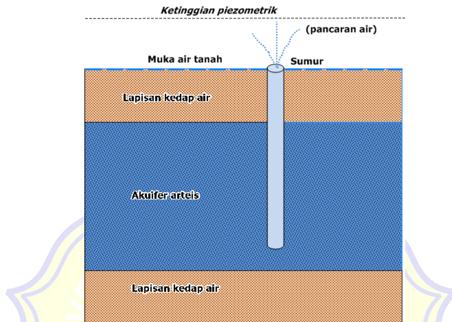
Gambar 1.1. Struktur Air
