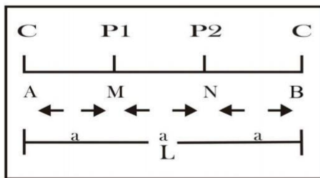
Gambar 2.5 Susunan elektroda arus dan potensial pada konfigurasi Wenner (Loke, M.H, 2004).
