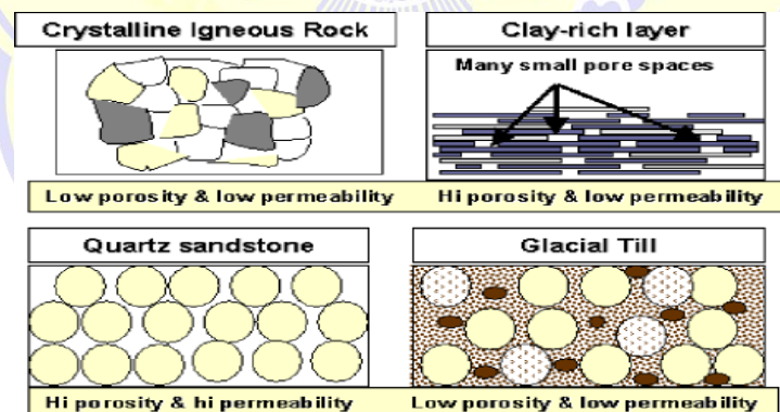
Gambar 2.2. Porositas dan Permeabilitas (Seyhan, 1977).
