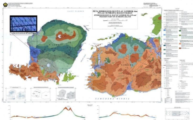
Gambar 2.7 Peta Hidrogeologi Pulau Lombok (Sudadi, 2000)
