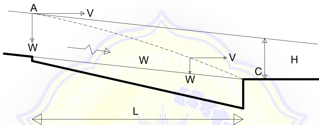
Gambar 2.8 a Potongan Memanjang Kantong Lumpur
