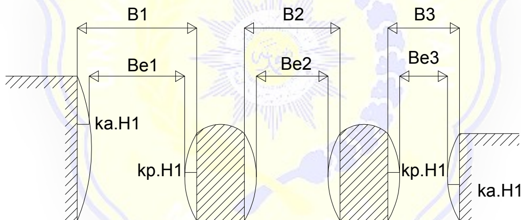
Gambar 2.10 Sketsa Lebar Efektif Bendung
