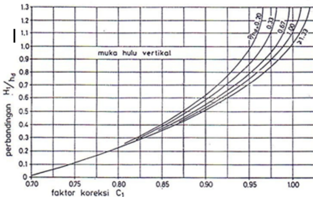
Gambar 2.18 Faktor Koreksi untuk Selain Tinggi Energi Rencana pada Bendung Mercu Ogee (Menurut Ven Te Chow, 1959, Berdasarkan Data USBR dan WES)
