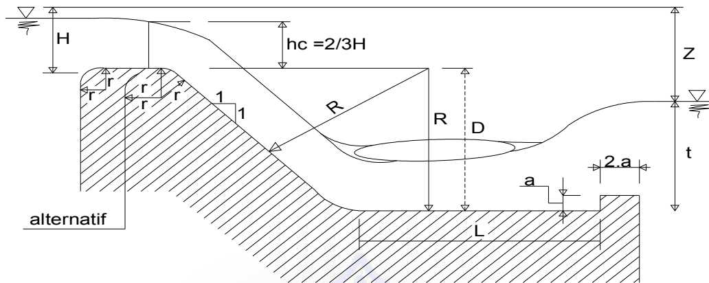
Gambar 2.21 Kolam Vlughter
