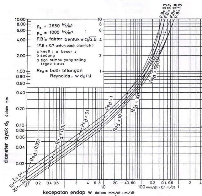
Gambar 2.9 Grafik Hubungan Diameter Saringan dan Kecepatan Endap Lumpur untuk Air Tenang
