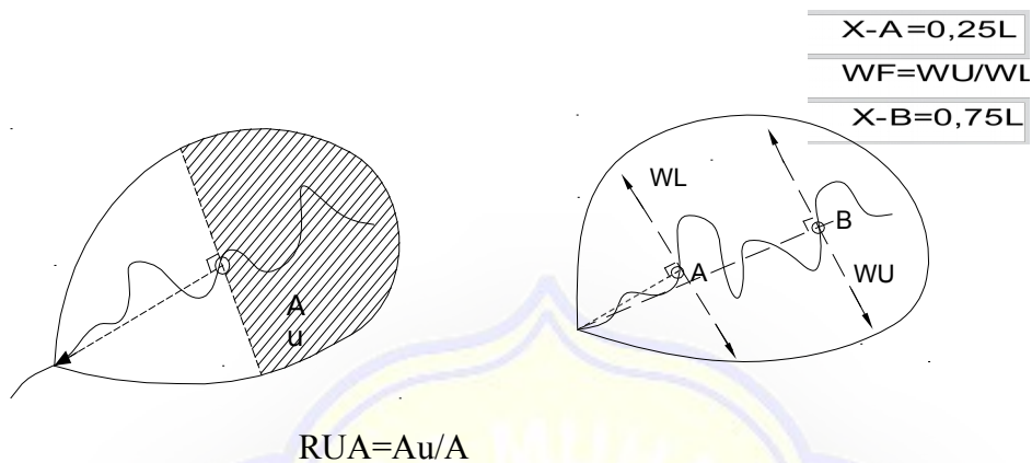
Gambar 2.4. Sketsa Penetapan RUA
