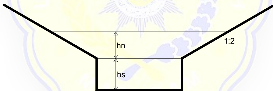
Gambar 2.8 b Potongan Melintang Kantong Lumpur
