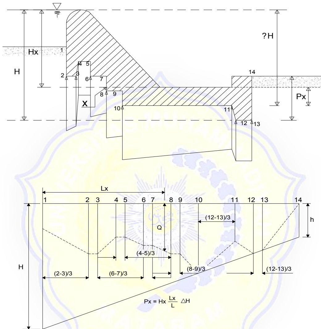
Gambar 2.23 Gaya Angkat pada Pondasi Bendung
