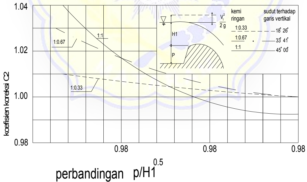
Gambar 2.15 Harga-harga Koefisien C_2 untuk Bendung Mercuri Ogee dengan Muka Hulu Melengkung (menurut USBR,1960)
