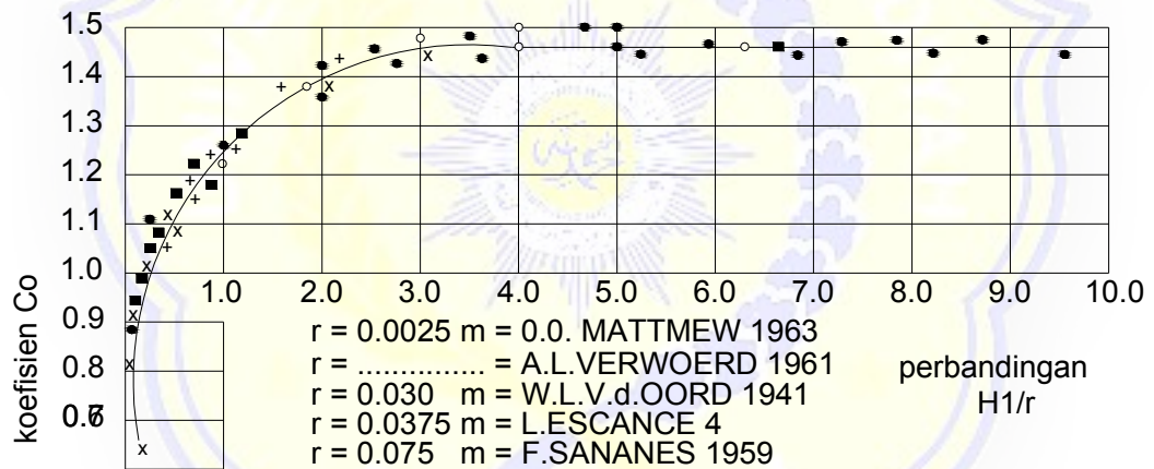
Gambar 2.13 Harga-harga Koefisien C_0 untuk Bendung Ambang Bulat sebagai Fungsi Perbandingan H_1/r (Sumber : KP-02 Bangunan Utama)
