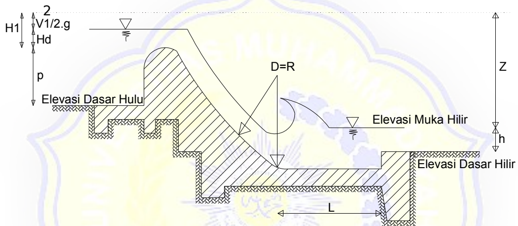
Gambar 2.19 Elevasi Air di Hulu dan Hilir Bendung
