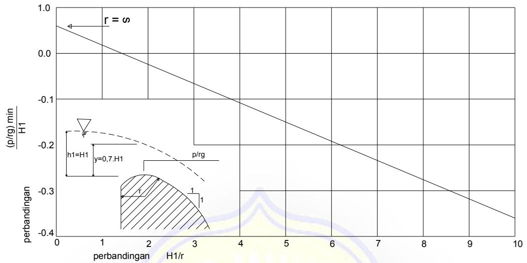
Gambar 2.12 Tekanan pada Mercu Bendung Bulat sebagai Fungsi Perbandingan H_1/r (Sumber : KP-02 Bangunan Utama)
