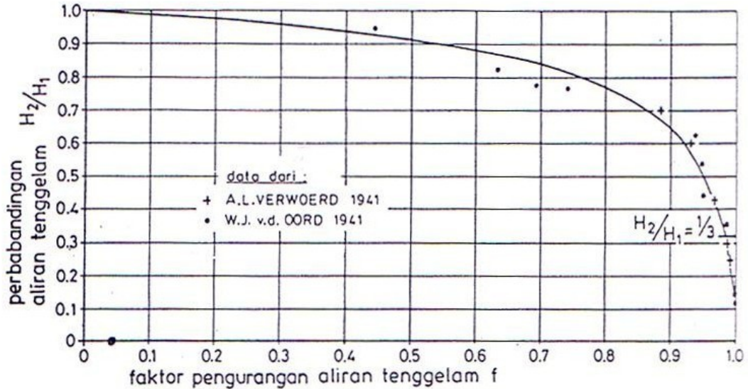
Gambar 2 16 Faktor Pengurangan Aliran Tenggelam sebagai Fungsi H_2/H_1
