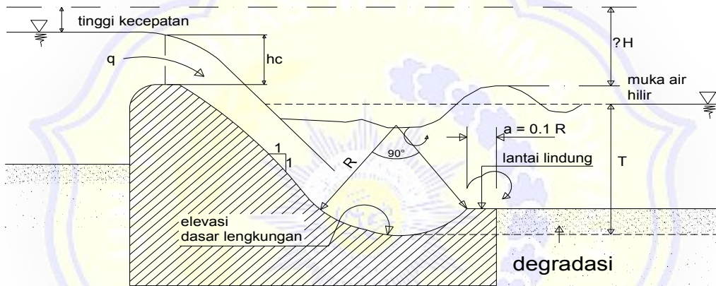
Gambar 2.20 Kolam Olak Tipe Bak Tenggelam
