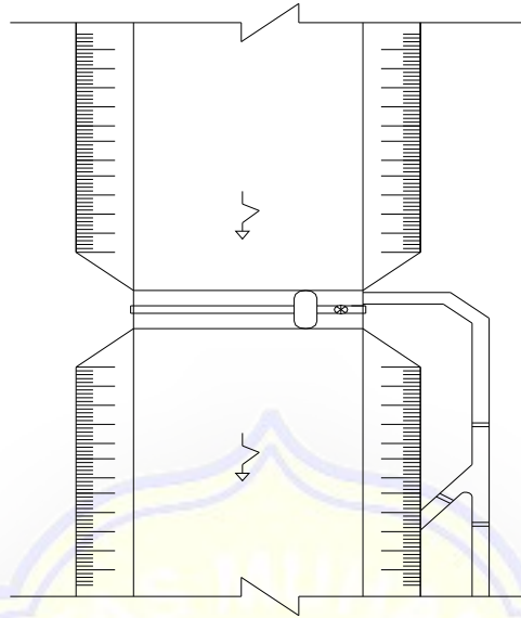
Gambar 2.5 Skema Bendung Tetap, Intake Kiri dengan Kantong Lumpur.
