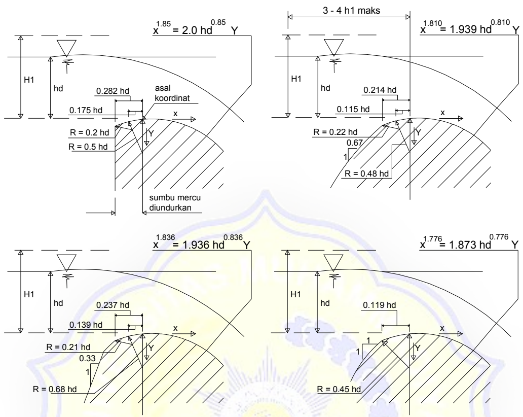
Gambar 2.17 Tipe Mercu Ogee
