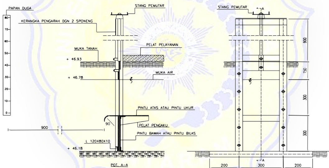
Gambar 2.7 Alat Ukur Romijn
