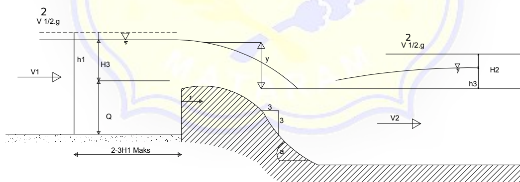
Gambar 2.11 Bendung dengan Mercu Bulat
